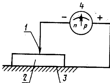
1 — зонд; 2 — образец; 3 — металлическая пластина; 4 — нуль-индикатор
